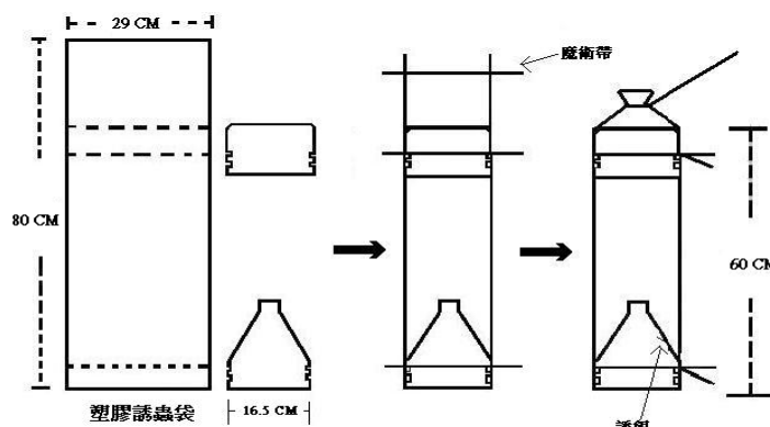
黑角舞蛾上衝式誘蟲器組裝流程圖
